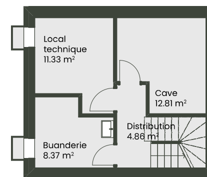
SOUS-SOL
