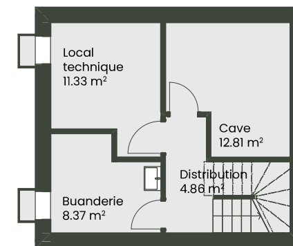
SOUS-SOL
